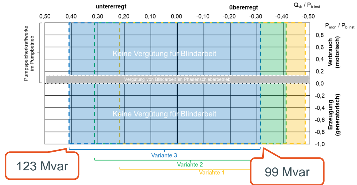
Beispielhafte Darstellung für Typ 1 Erzeugungsanlagen
